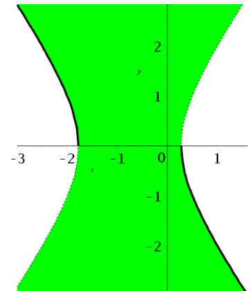
Рис. 2. Розв'язки нерівності 3z^2 + 2z + 1 < 0
