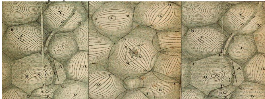
Рис. 1. Прообраз діаграм Вороного у роботі Рене Декарта.
